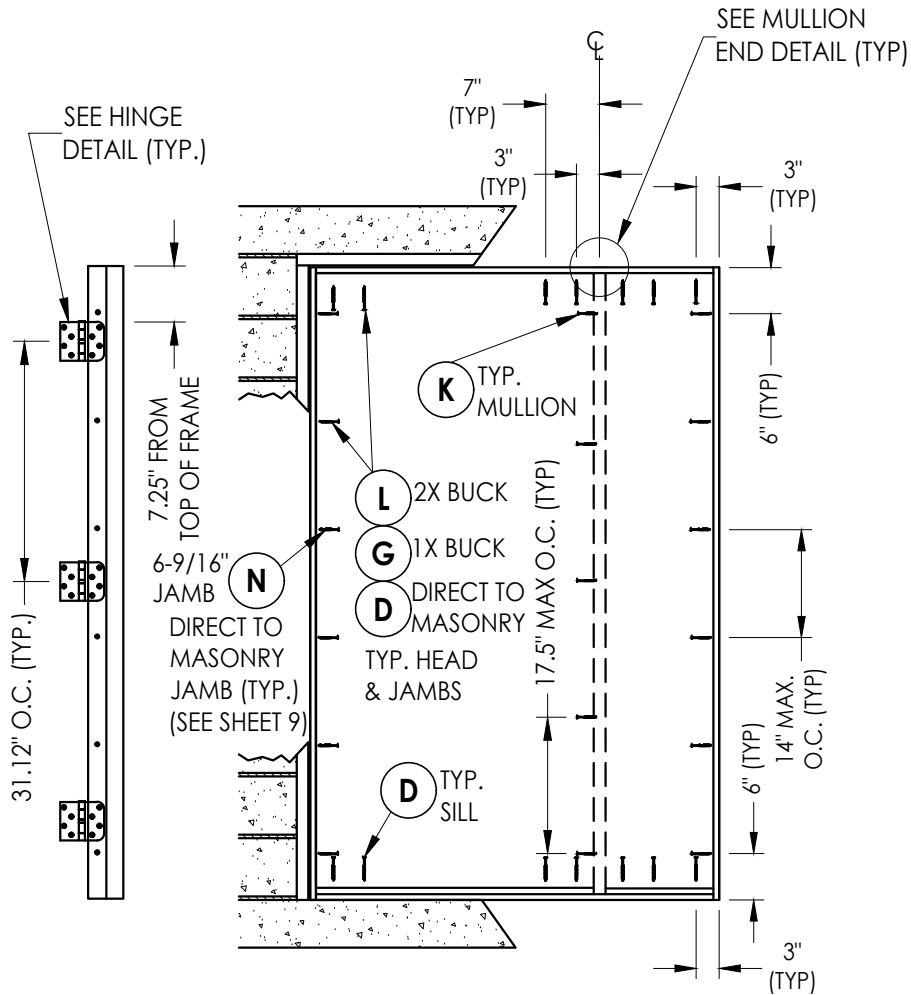
HINGE JAMB
